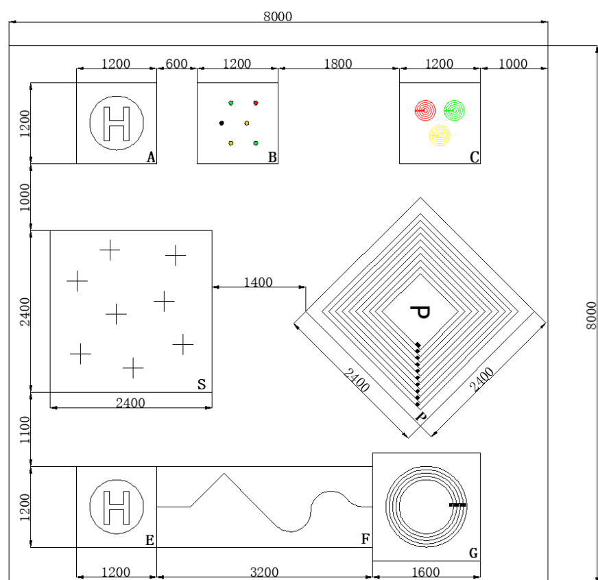
图 2: 场地尺寸图
